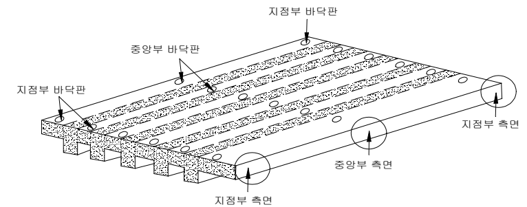
【그림 3.2.1】콘크리트 바닥판 조사부위에 따른 손상종류
