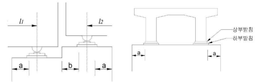
(a) 선로방향
