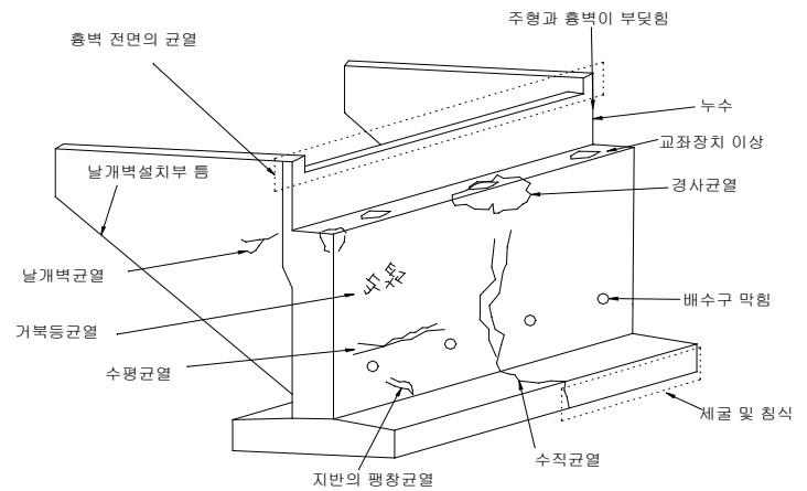
【그림 3.2.11】 교대의 조사부위
