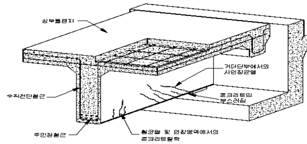
【그림 3.2.5】 철근콘크리트 거더의 조사부위
