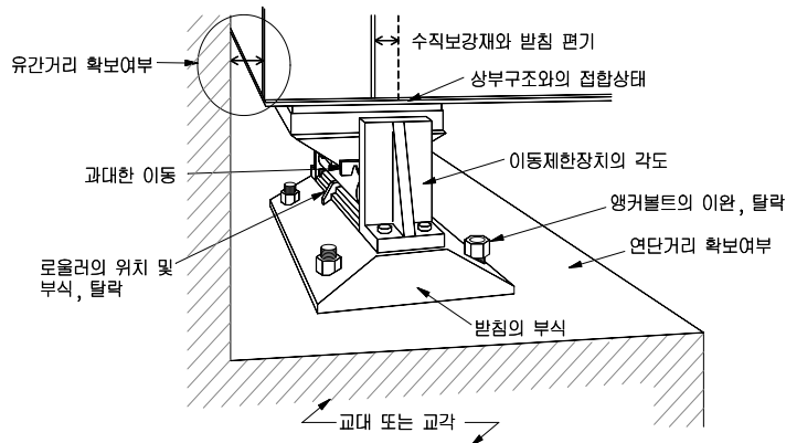
【그림 3.2.16】교량받침 조사부위
