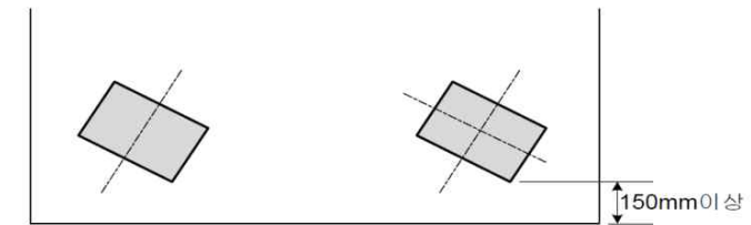
【그림 3.2.19】 사각을 가진 거더에서 받침의 배치
