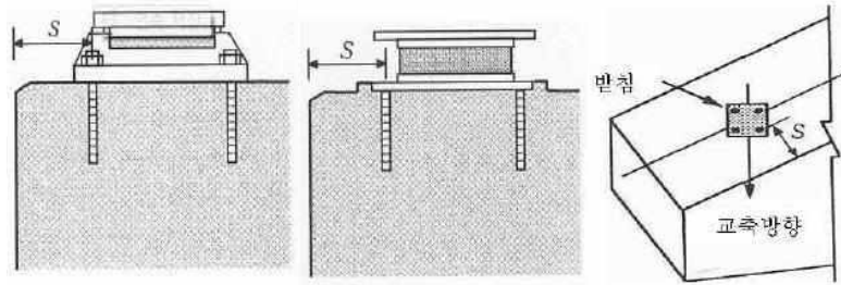
【그림 3.2.17】 교량받침 연단거리
