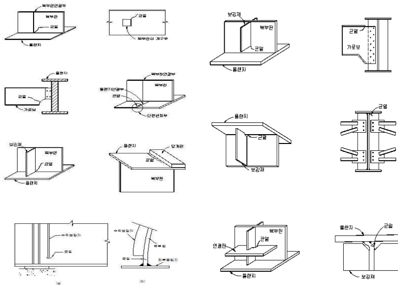
【그림 3.2.3】 피로균열이 발생하기 쉬운 구조상세
