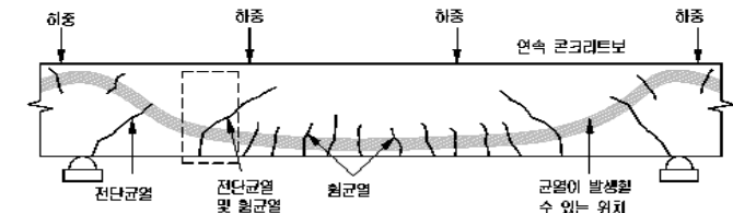
【그림 3.2.4】 콘크리트 거더에 발생하는 균열의 유형과 위치
