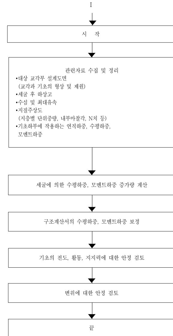
【그림 4.1.2】 2단계 기초안전성 평가결과 산정 방법
