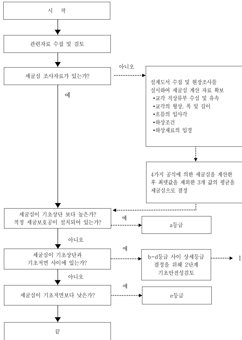
【그림 4.1.1】 1단계 세굴심 평가결과 산정 방법
