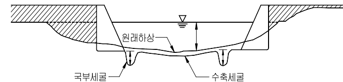
【그림 3.2.14】 수축세굴과 국부세굴
