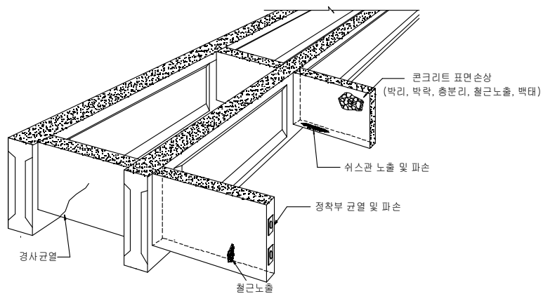
【그림 3.2.7】 콘크리트 가로보 조사부위 및 조사사항
