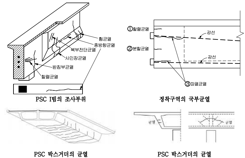
【그림 3.2.6】 프리스트레스트 거더별 조사부위 및 균열
