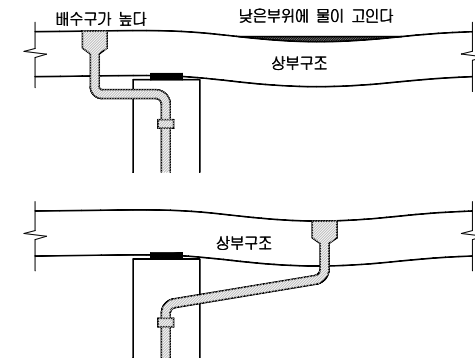
【그림 3.2.21】 배수구 물고임
