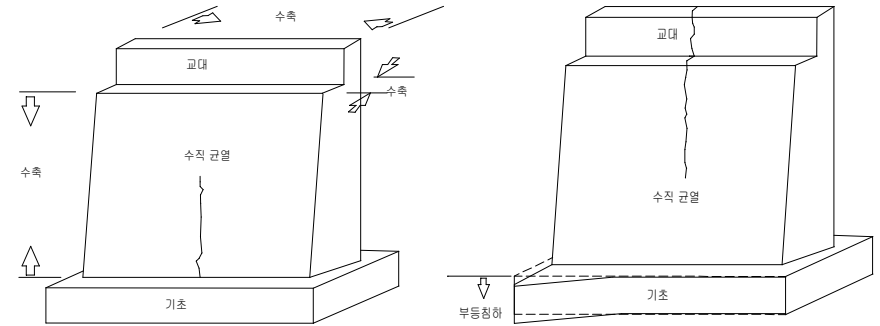
【그림 3.2.9】 온도응력, 건조수축에 의한 교대의 수직균열
