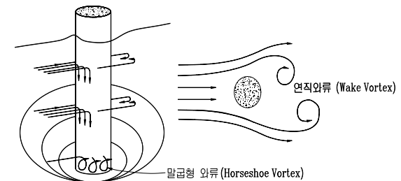
【그림 3.2.15】 원형기초의 국부세굴
