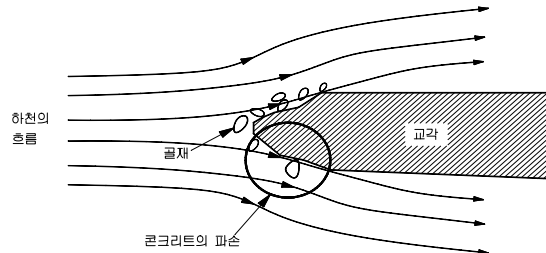
【그림 3.2.13】 유수에 의한 콘크리트 교각의 침식
