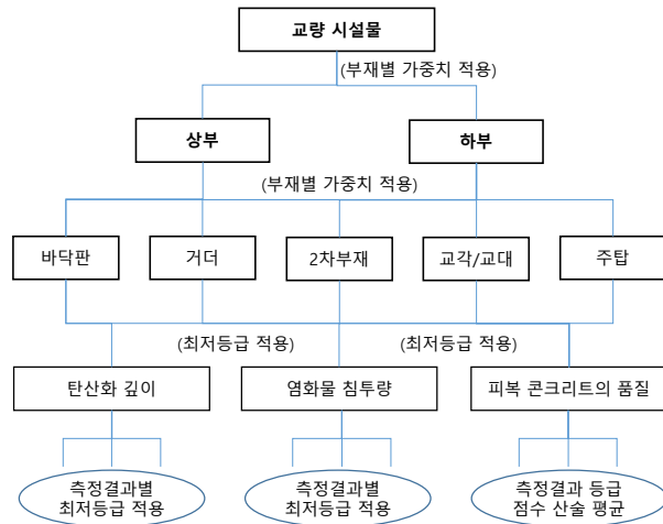
【그림 4.2.2】콘크리트 내구성능 항목별 세부 평가방법
