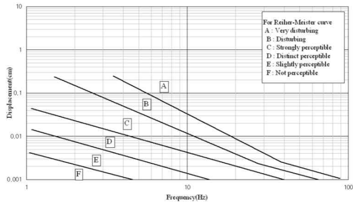
【그림 4.3.1】Reiher-Meister(1931)의 허용곡선
