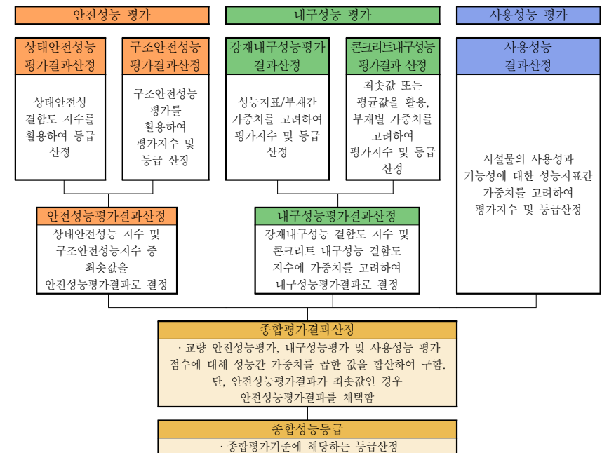
【그림 4.4.1】 교량의 종합성능등급 지정 절차
