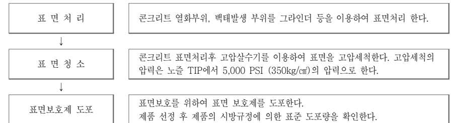
【그림 5.3.1】 콘크리트 표면처리 시공순서도
