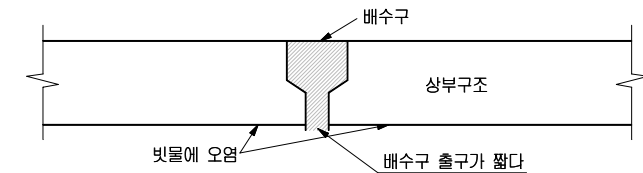
【그림 3.2.22】 배수구 길이 부족
