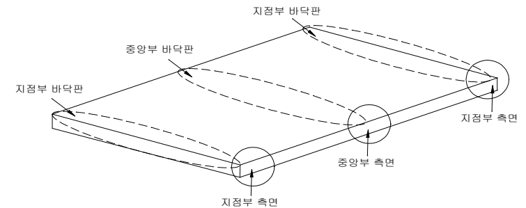
【그림 3.2.2】거더가 없는 경우의 바닥판 조사부위
