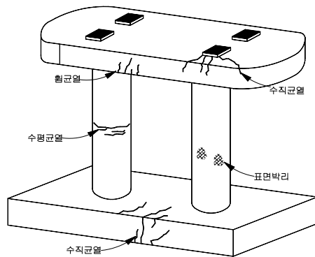
【그림 3.2.12】 콘크리트 교각의 조사부위
