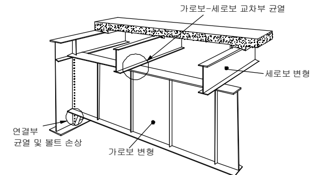
【그림 3.2.8】 강가로보, 강세로보의 조사부위 및 조사사항
