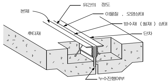
【그림 3.2.20】 신축이음 조사부위
