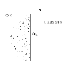
【그림 5.3.3】 표면처리 보수공법 개요도
