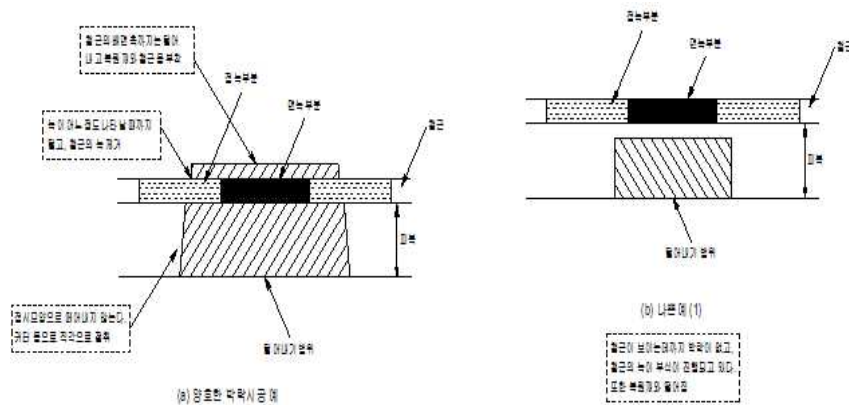
【그림 5.3.4】 단면복구(보수) 상세도
